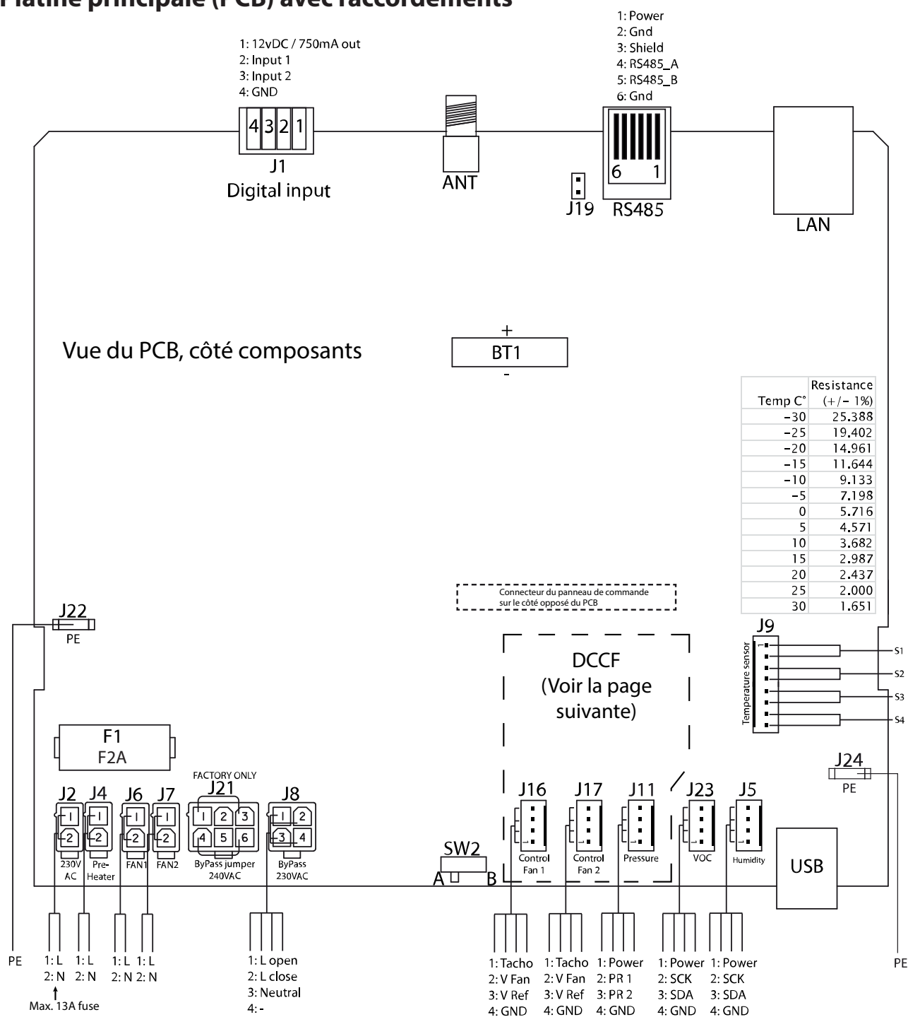
Fig. 62 : Platine principale (PCB) avec raccords
