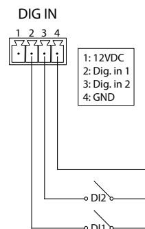
Fig. 22: Digital indgang
