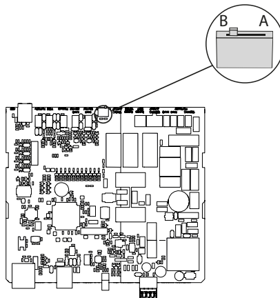
Afb. 45: Bedrijfsmodus controleren
