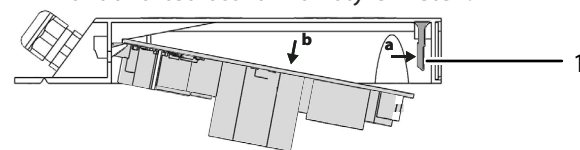
Fig. 29: Lossa huvudkortet
