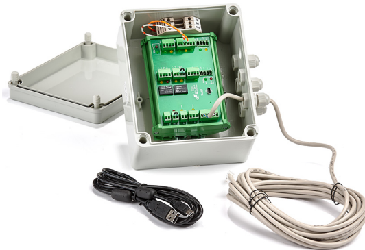
Fig. 16: Ekstra styreenhed HAC 2
