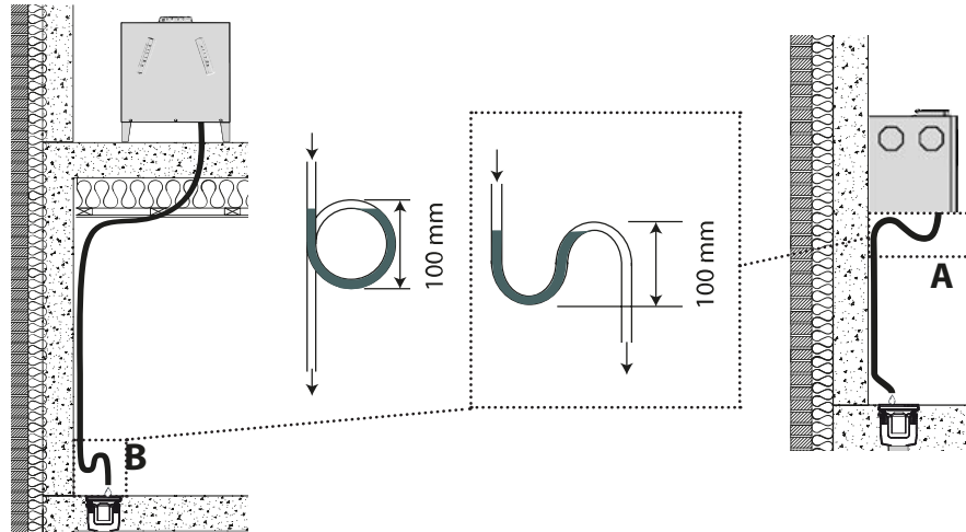
Afb. 49: Sifon maken
