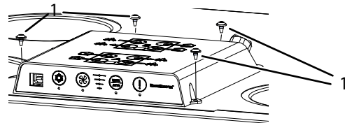
Fig. 26: Demontera skruvarna
