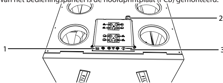
Afb. 20: Bedieningspaneel
