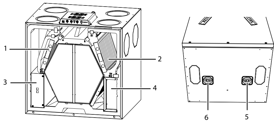
Fig. 11 : Sous-ensemble en mode A/B
