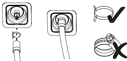
Afb. 47: Condensafvoerslang aansluiten
