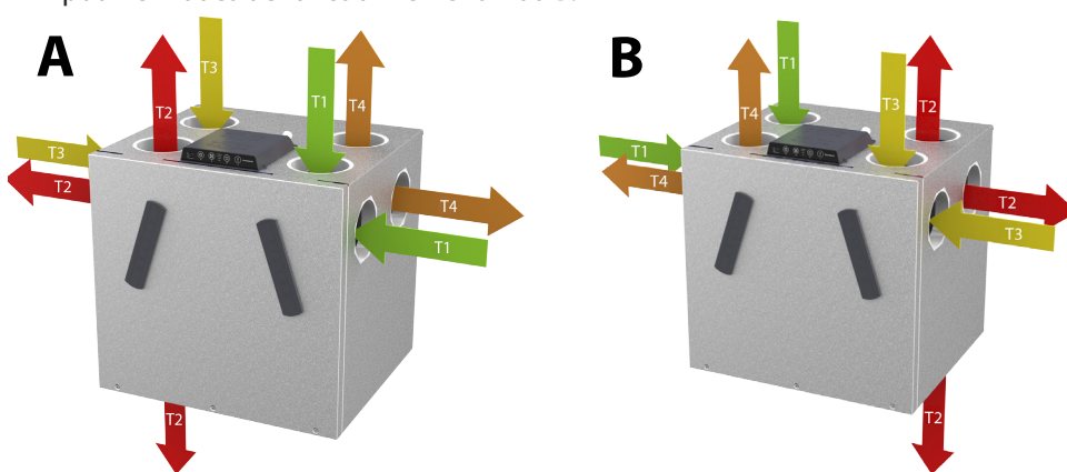
Fig. 51 : Observer les raccords
