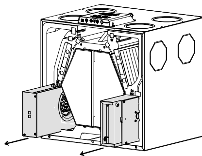
Abb. 58: Ventilatorgehäuse entnehmen
