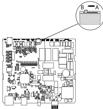
Fig. 31: Ställ omkopplaren i driftläge B
