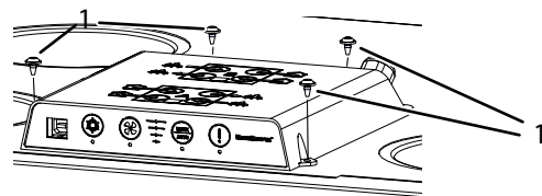
Afb. 26: Schroeven demonteren
