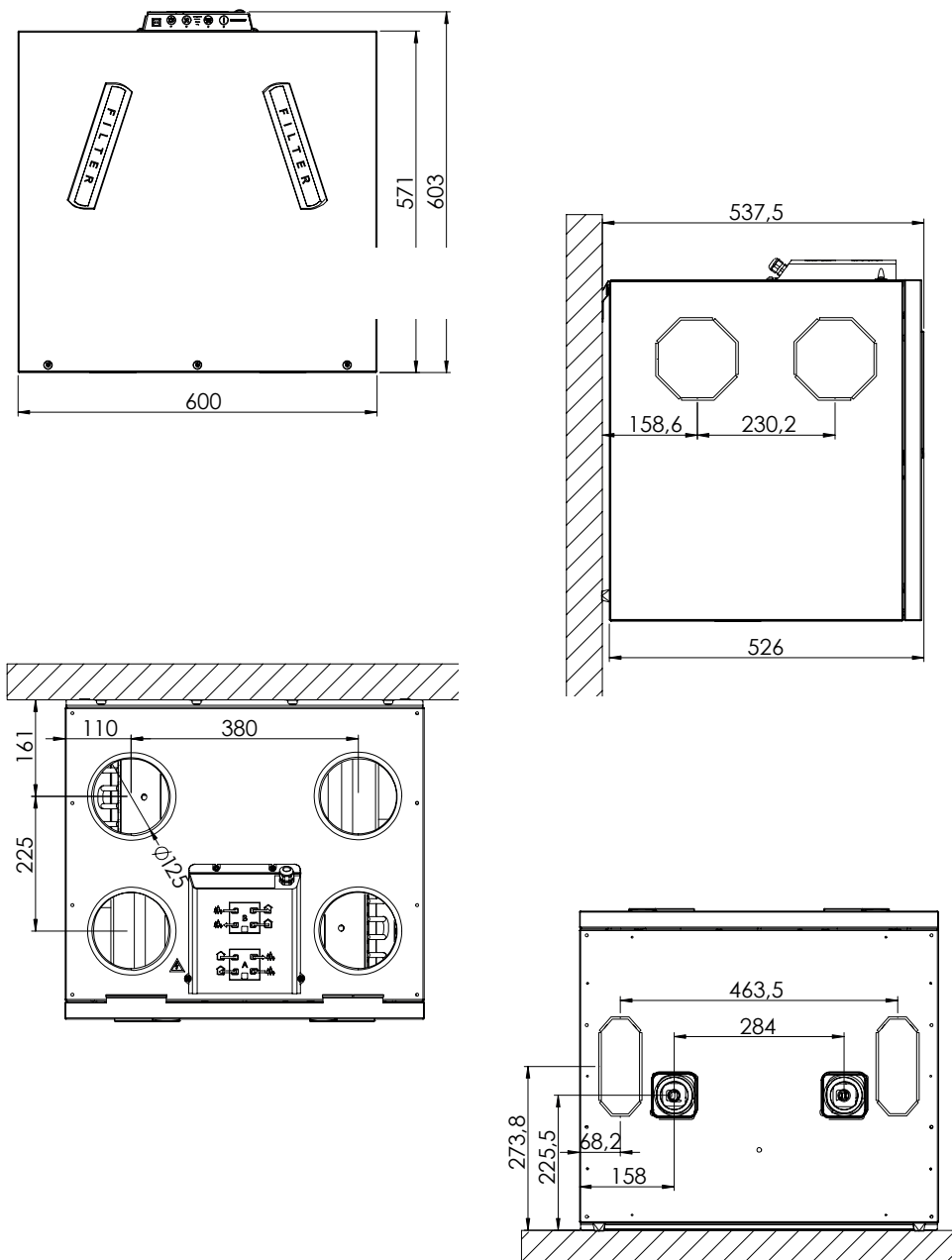
Fig. 60: Skåpmått
