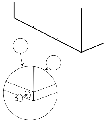
Fig. 40: Montera distanshållare
