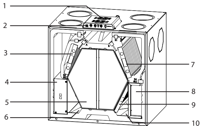
Fig. 8: RCV320/480/640 uden afdækning
