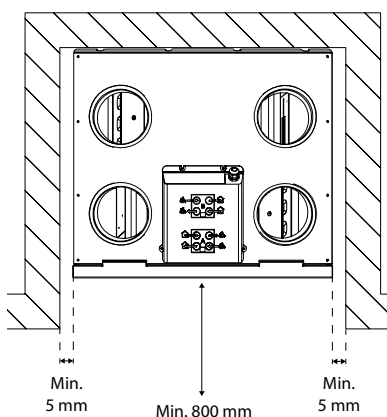
Fig. 23: Utrymmesbehov för underhållsaktiviteter
