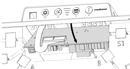
Sl. 30: Odstranitev plošče tiskanega vezja
