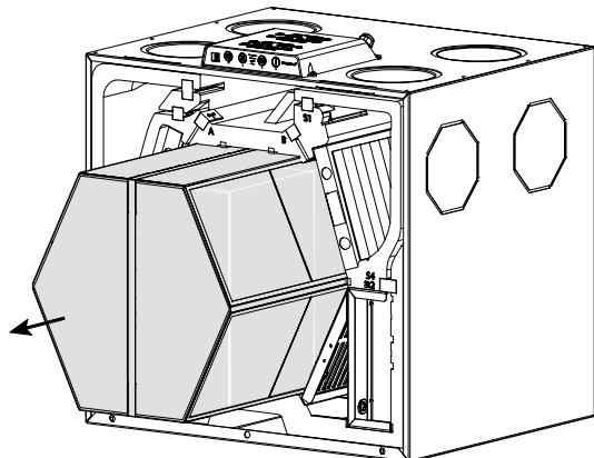
Abb. 59: Wärmetauscher entnehmen
