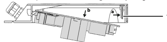
Fig. 29: Hovedprintkort løsnes
