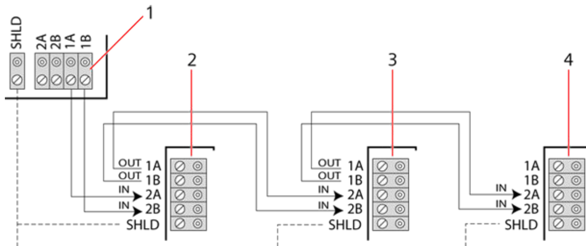
Streng-konfiguration
