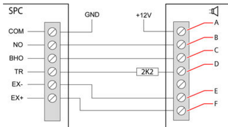
Ledningsføring af ekstern sirene
