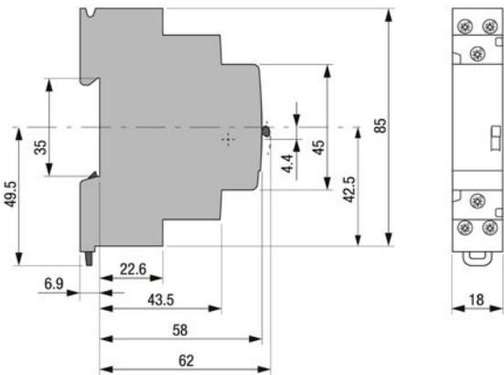
Stromstoßschalter E290
