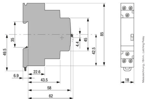
Zentral Ein-Aus Kontrollmodul E294 (für unterschiedliches Steuerspannungs-Potential)
