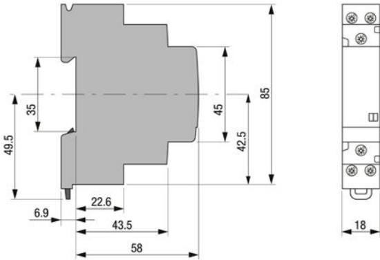
Sequentieller Stromstoßschalter E291S
