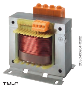
TM-C
