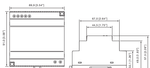
CP-D 24/4.2
