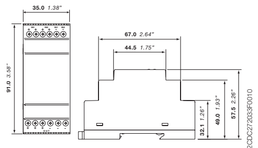
CP-D RU
