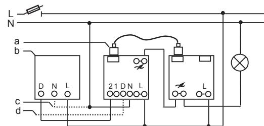
Busch Jäger 6592 U STD-500U STD-420E
