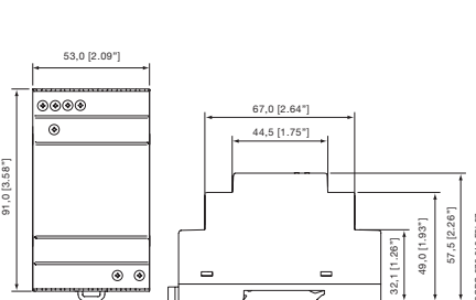
CP-D 12/2.1, CP-D 24/1.3
