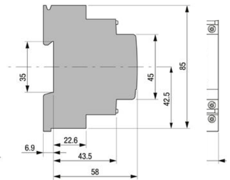
Hilfskontakt 11/-20
