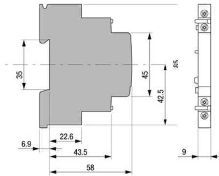
Hauptkontaktmodul E298
