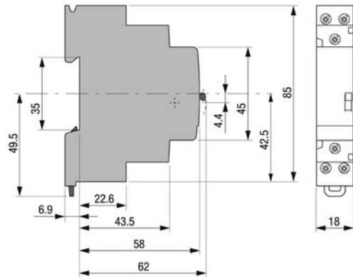
Installationrelais E297
