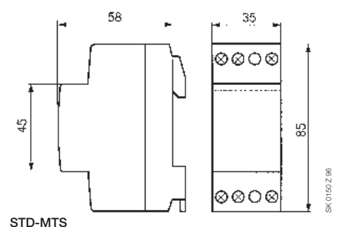
STD-MTS
