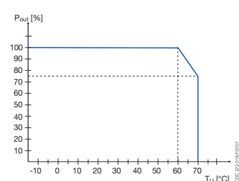
CP-D 24/2.5
