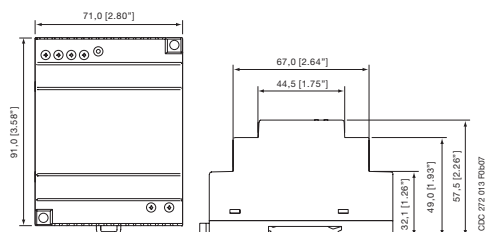
CP-D 24/2.5
