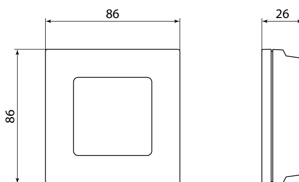
Trådløs termostat Danfoss lcon™
