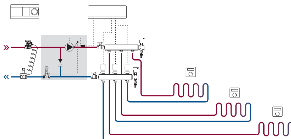
Eksempel 2: 2-rørsystem med gulvvarmeshunt (fremløbstemperaturregulering, ekstraudstyr)
