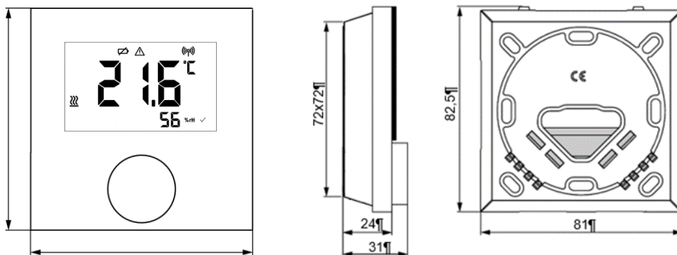
Fig. 1: Dimensioner på digital rumtermostat (i mm)
