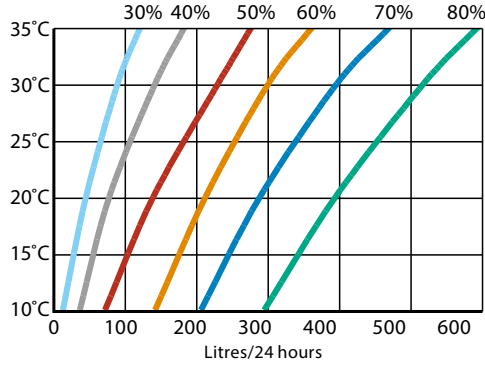
Ydelsesdata DH 300
