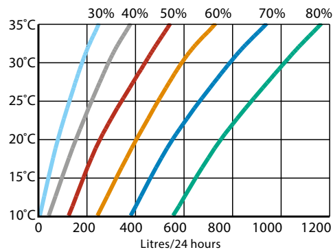
Ydelsesdata DH 600
