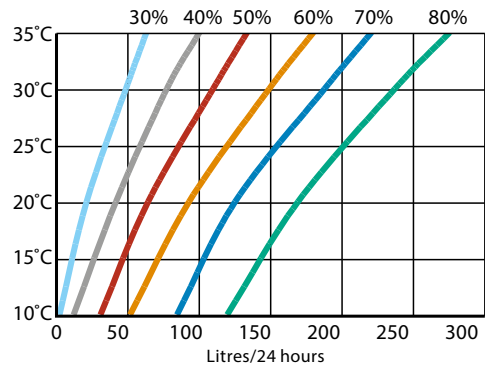
Ydelsesdata DH 150
