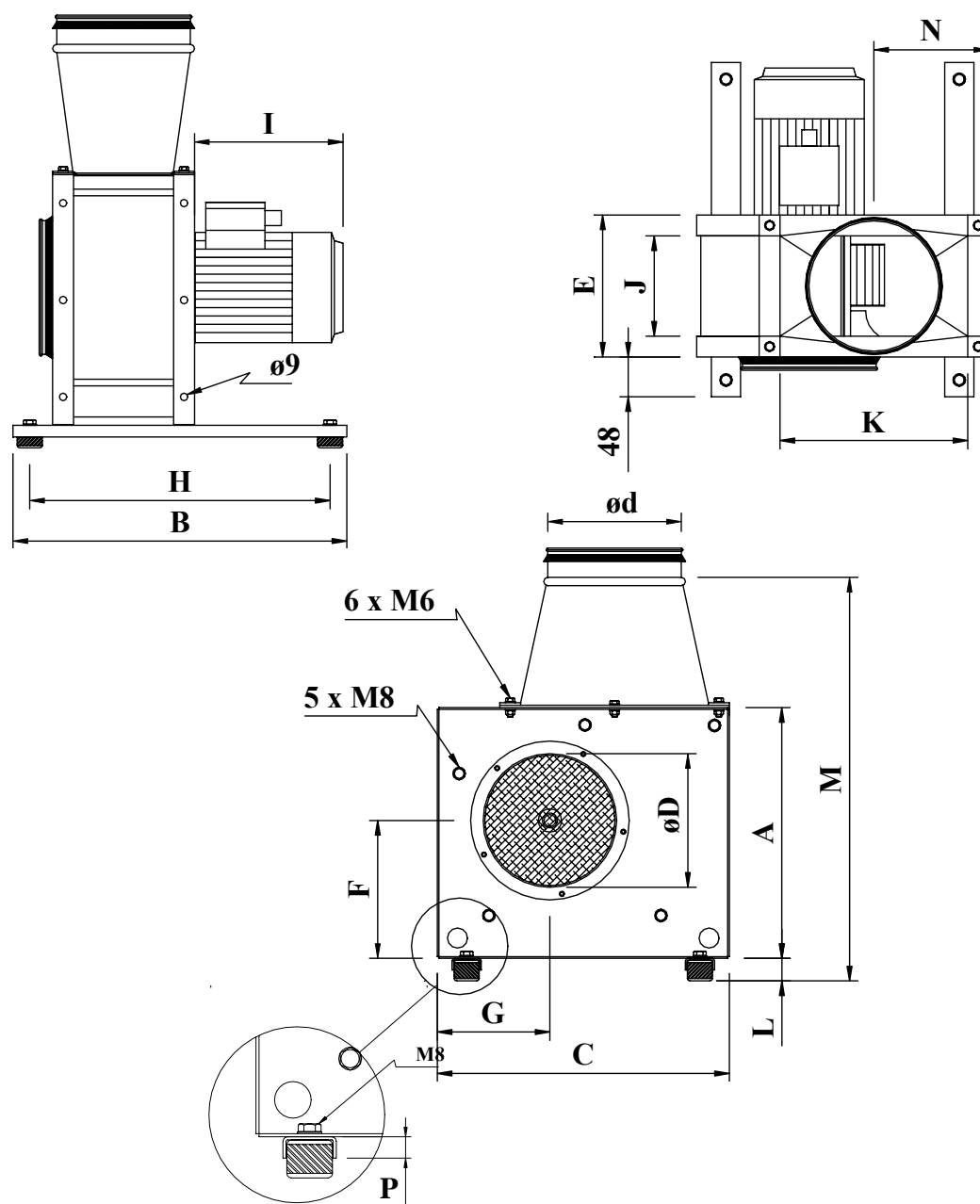
Måltabel, ventilatorer LEF/MEF (LEX/MEX)
