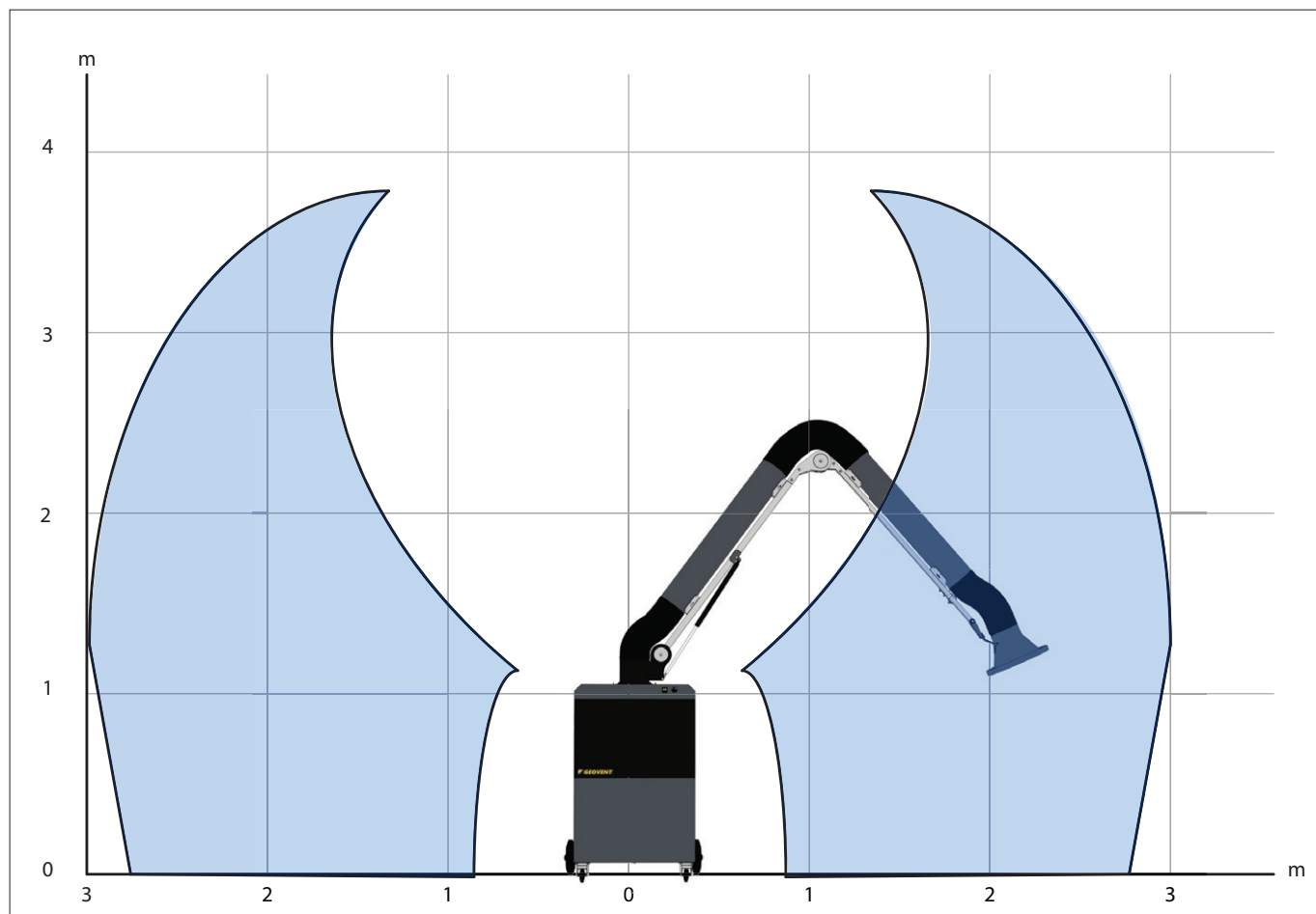
Arbejdsområde for GeoGo med ASA4 arm
