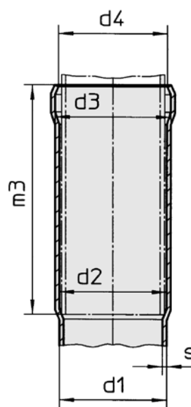
Tredobbelt muffe 3A Lang muffe 3A
