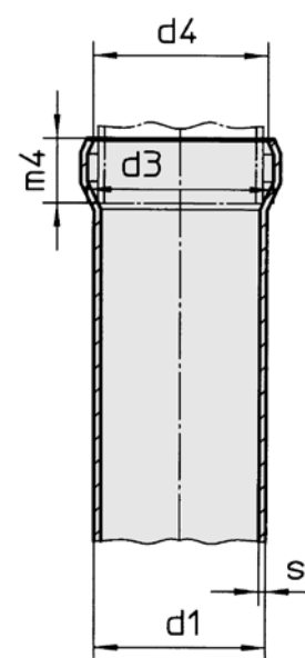
Kort muffe 4A Kort muffe 0,5A
