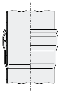
GM-X Push-fit-overgangsstykke Muffe DN 40-200 med tætningsring
