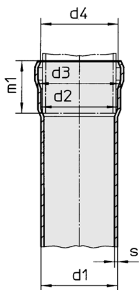
DIN 19530 Standardmuffe 1A EN 1123 Standardmuffe 1A
