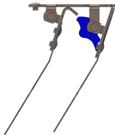
Spjæld-system til TX11 LOCK.
