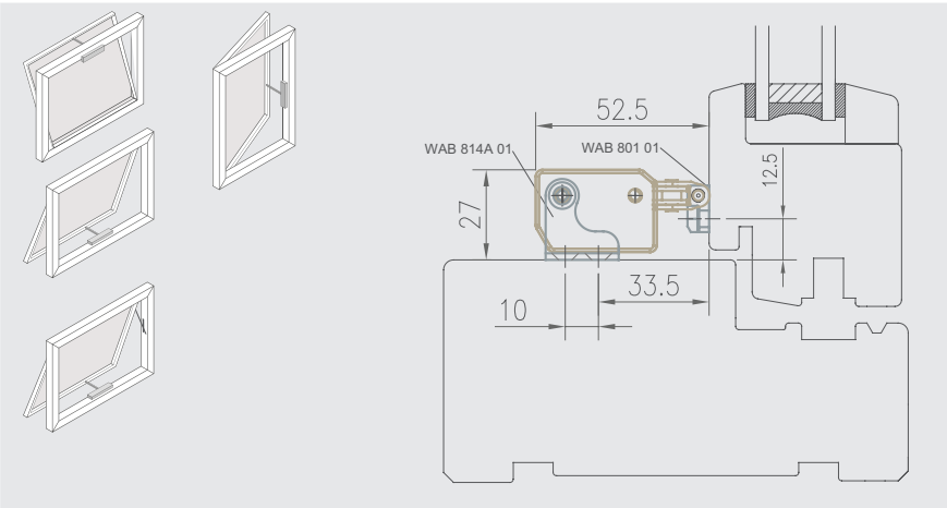
Montageforslag 5 - Udadgående vindue
