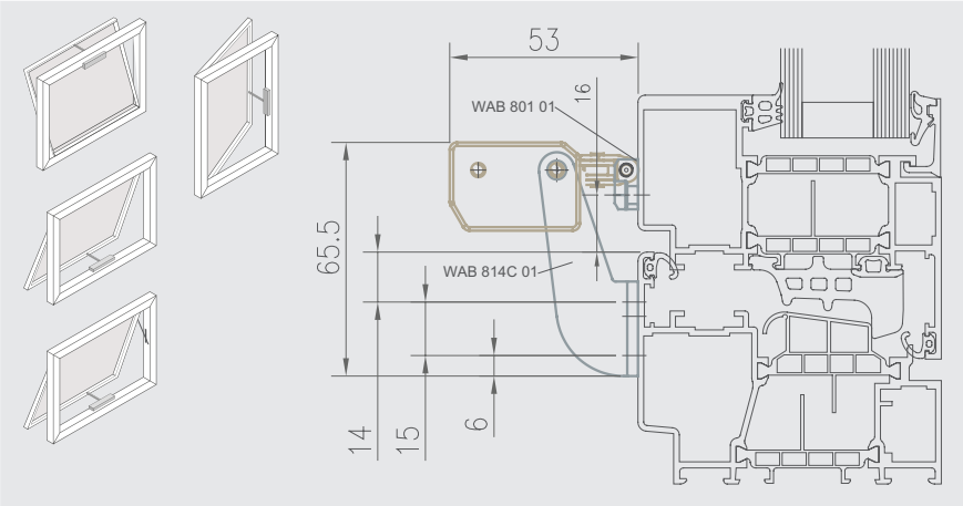
Montageforslag 4 - Udadgående vindue
