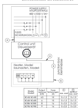
3-phase electrical connections of control unit C150 and BC-E heater 3-phasescher Elektroanschlüsse des Steuergeräts C150 und des Saunaofens BC-E
