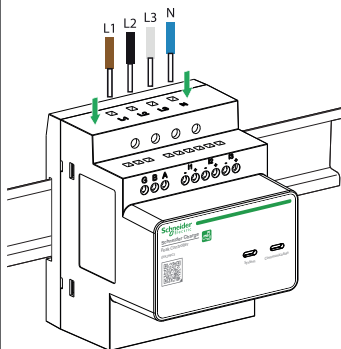
230V AC 3-fases
