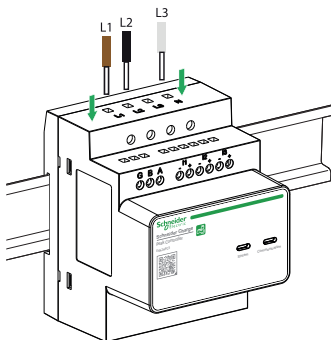
230V AC 3-Phasen Kein Neutraleiter
