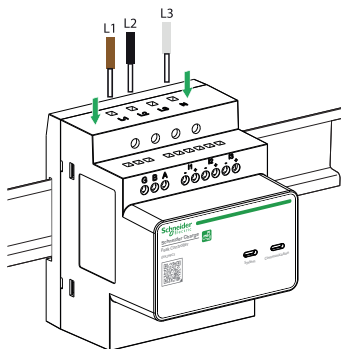
230V AC 3-fases no neutral
