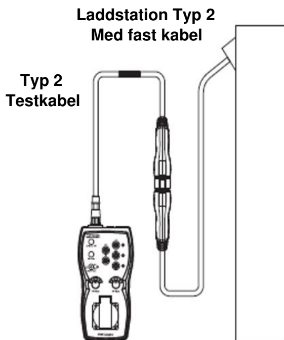
Anslutning av testadaptern till en laddstation typ 2 med fast kabel och fordonsuttag
