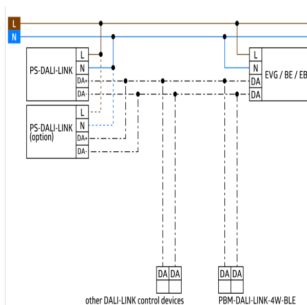
Ledningsdiagram
