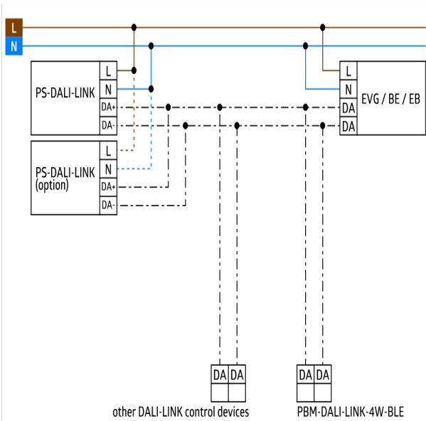
Ledningsdiagram
