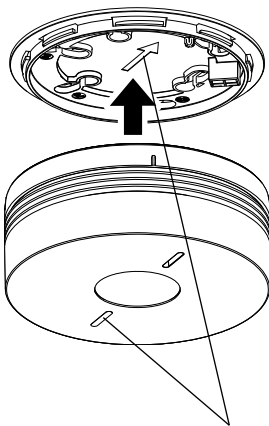
Ausrichtung des Melders an der Decke
