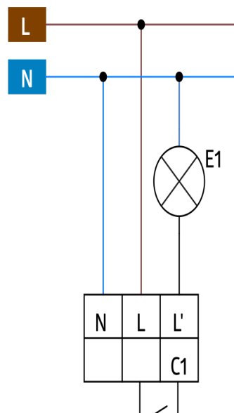
Ledningsdiagram
