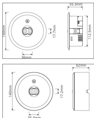
Dimensioner i mm
