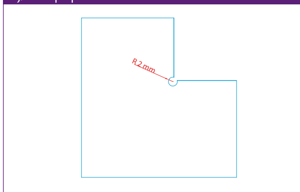
Hjørneklip i plade
