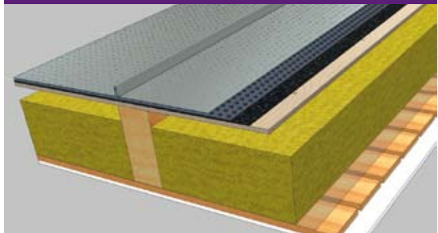
Konstruktion ved Ikke-kompatibelt underlag i kombination med lav taghældning (mindre end 35 grader)
