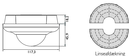
Fig. 3 - typenr. 41-701, 41-771
