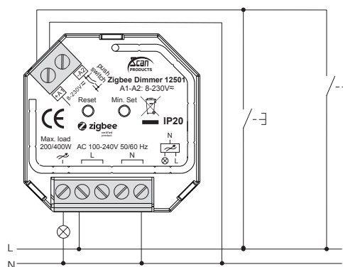
Ledningsdiagram
