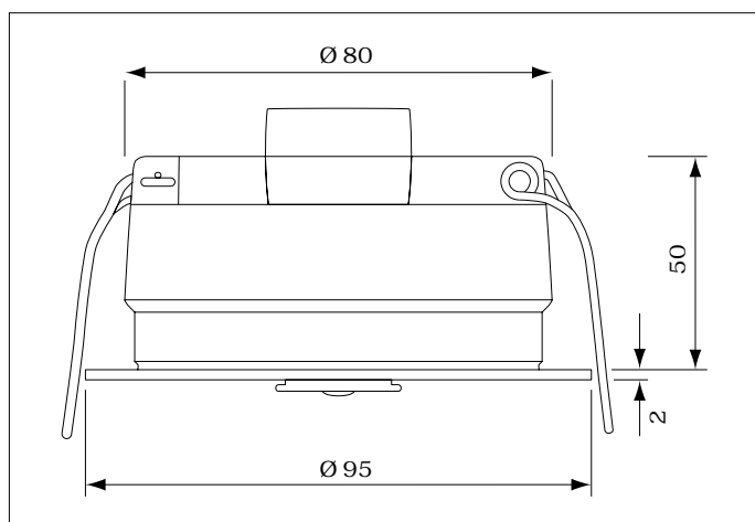
Dimensioner i mm
