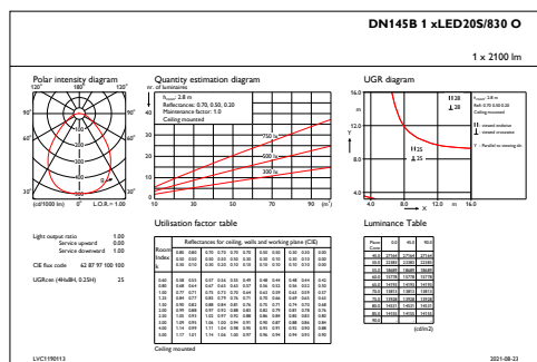
IFGU1_DN145B1xLED20S8300
