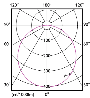
DN065B G4 LED12 830 12W D150 RD
