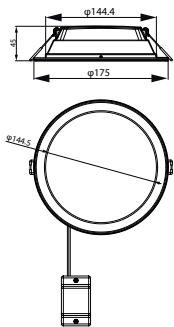
DN065B G4 LED12/830 12W 220-240V D150 RD
