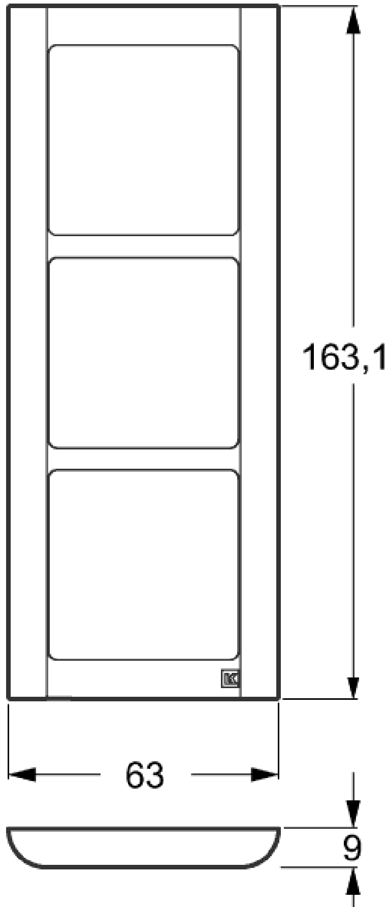
Målskise
