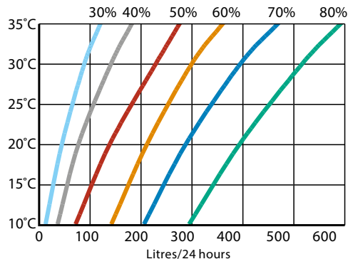
Ydelsesdata DH 300
