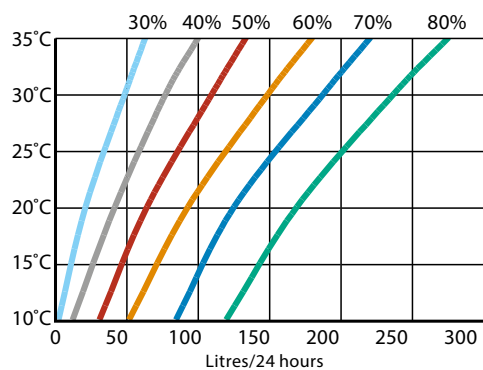
Ydelsesdata DH 150
