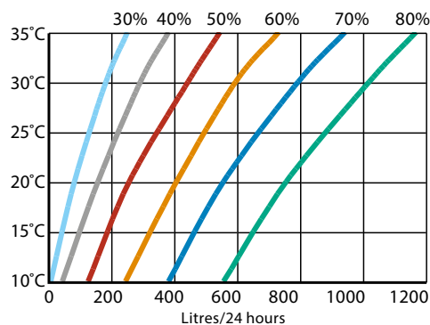
Ydelsesdata DH 600
