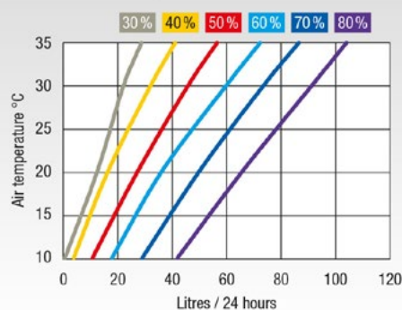
Dehumidification performance DH 60
