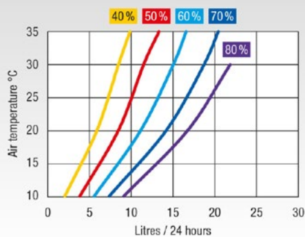
Dehumidification performance DH 15
