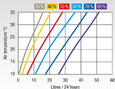
Dehumidification performance DH 30
