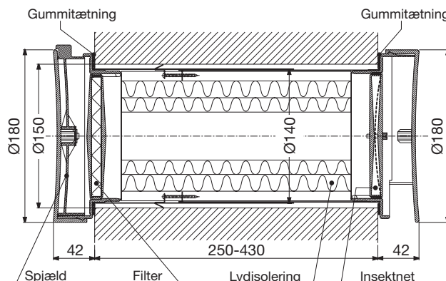
Udvendig rist type 1
