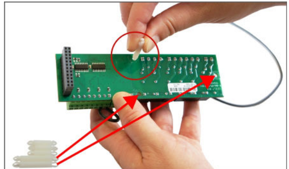
2. Monter de store af de medfølgende printkortholdere i de 3 huller på optionsprintet.
