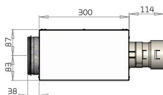
2 Stutse - Varenr. 8528204
