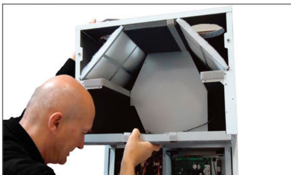
11. Toppen løftes af den nederste del.
