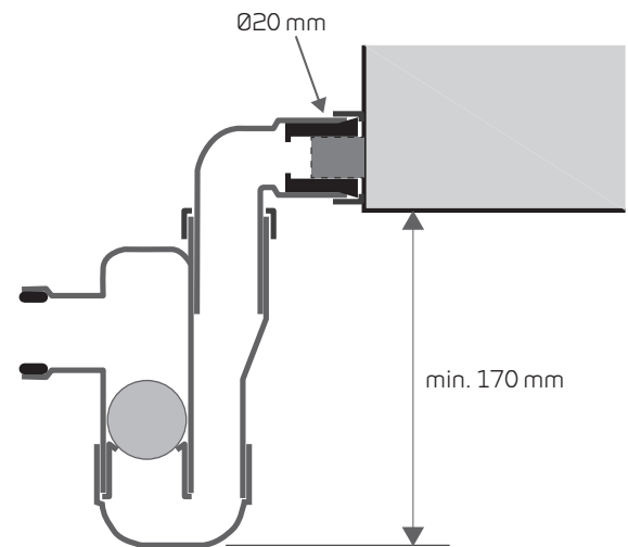
Tilslutning af Nilans vandlås med bold
