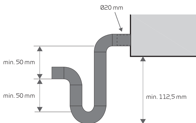
Tilslutning vandlås generelt
