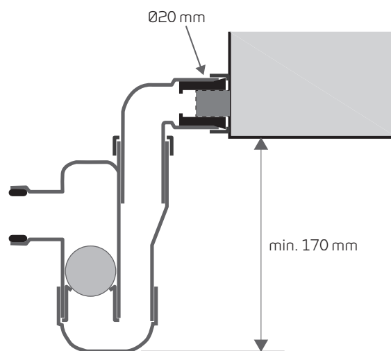
Tilslutning af Nilans vandlås med bold
