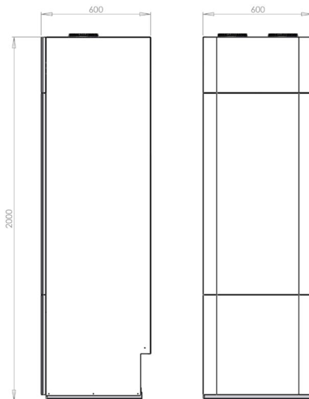
Figur 3: Ydre dimensioner
