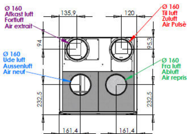
Figur 2: Kanaltilslutning
